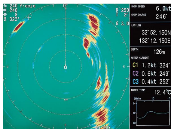
Imagem do monitor do Color Scanning Sonar CSH-5L, mostrando a embarcação no centro e cardumes de peixes nos entornos (registros vermelhos e amarelos).
